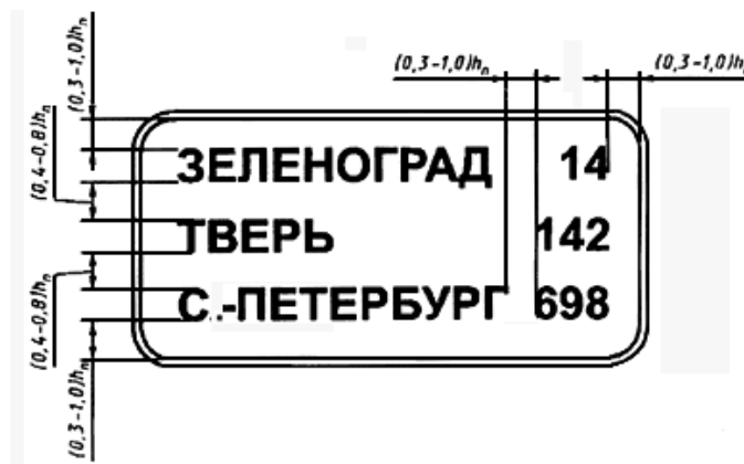
Рисунок Г.5 - Пример компоновки знака индивидуального проектирования 6.12
