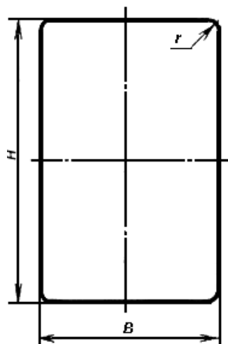
Рисунок Д.7 - Размеры прямоугольных знаков вертикального формата
