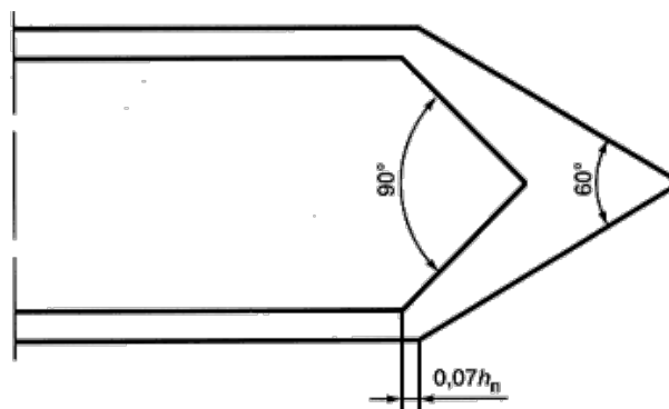
Рисунок Г.2 - Конфигурация оголовка знака индивидуального проектирования 6.10.2
