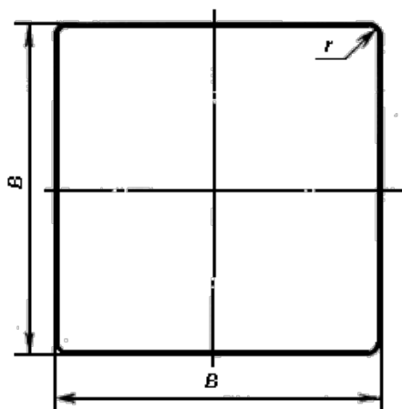
Рисунок Д.5 - Размеры квадратных знаков
