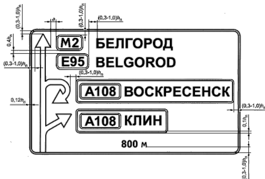
Рисунок Г.3 - Пример компоновки знака индивидуального проектирования 6.9.1
