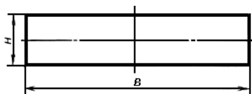
Рисунок Д.6 - Размеры знаков 1.34.1-1.34.3
