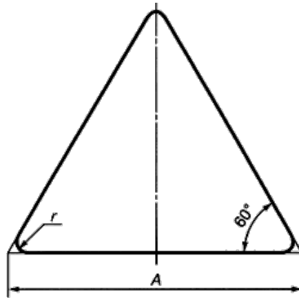
Рисунок Д.1 - Размеры треугольных знаков
